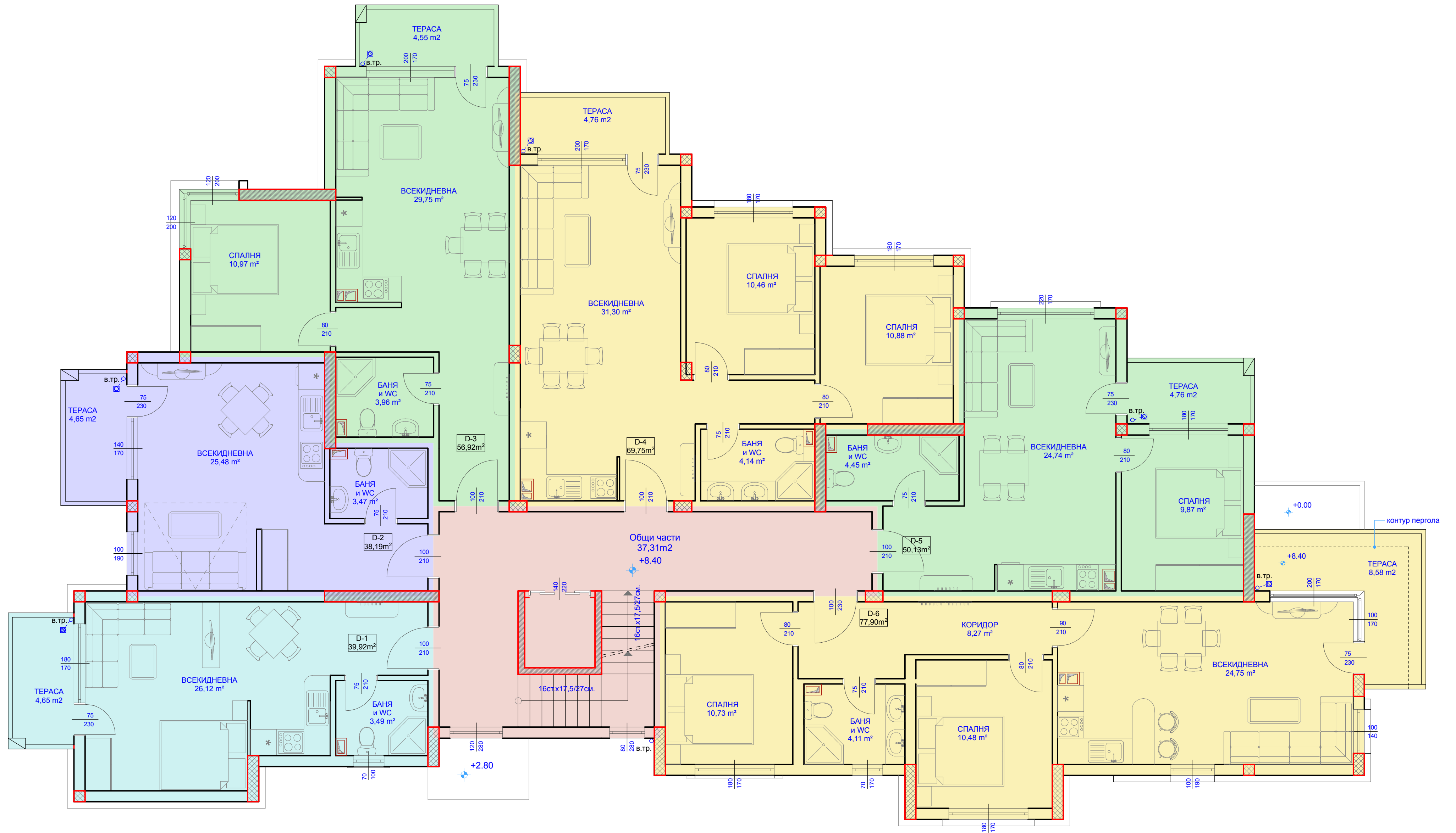
РАЗПРЕДЕЛЕНИЕ - КОТА +8.40
