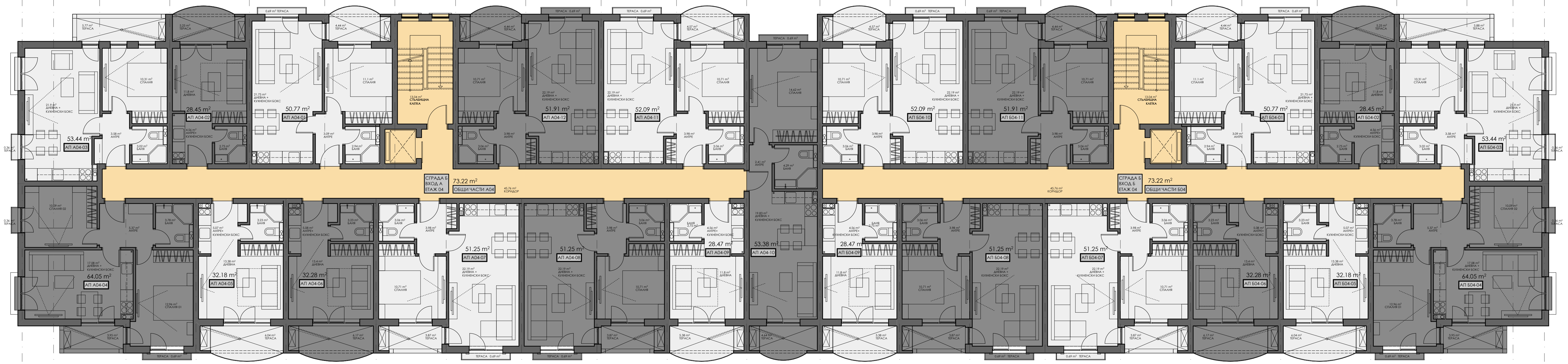
РАЗПРЕДЕЛЕНИЕ ЕТАЖ 04 1192.21m 2 СТРАДА Б
