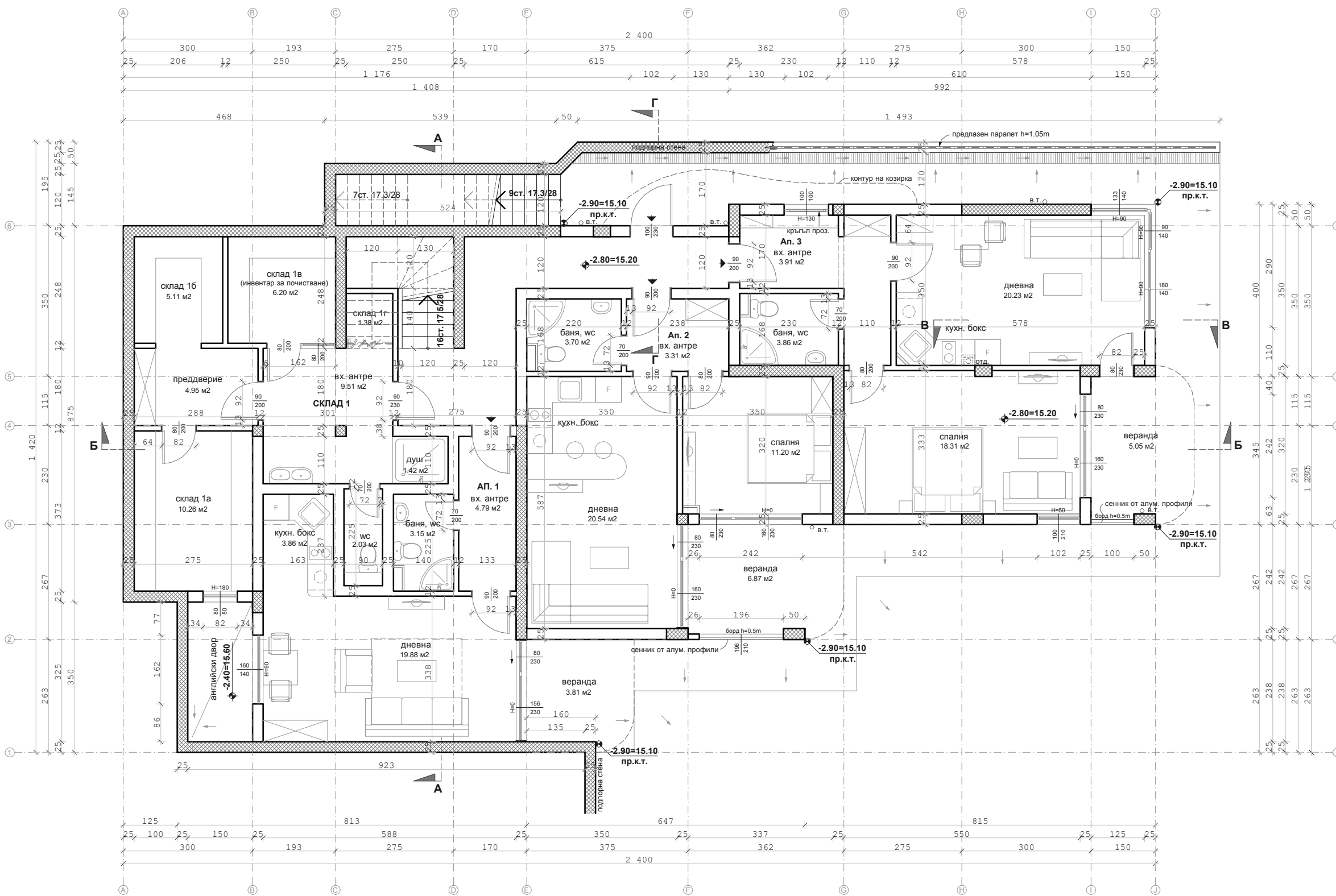
РАЗПРЕДЕЛЕНИЕ НА СУТЕРЕН (КОТА -2.80) Площ: 238.60 м2
